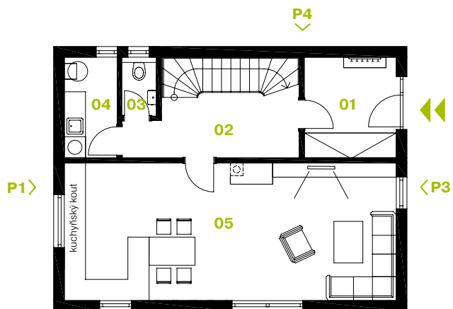
PŮDORYS PŘÍZEMÍ
