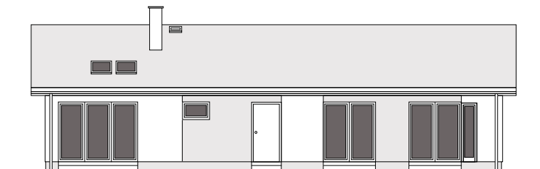
POHLED P1
