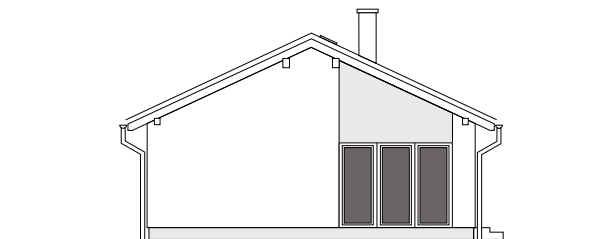
POHLED P2
