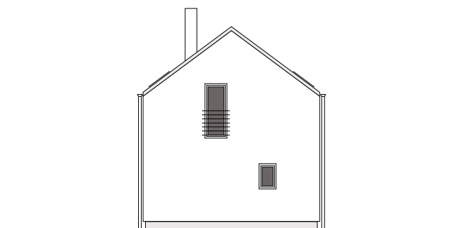
POHLED P2
