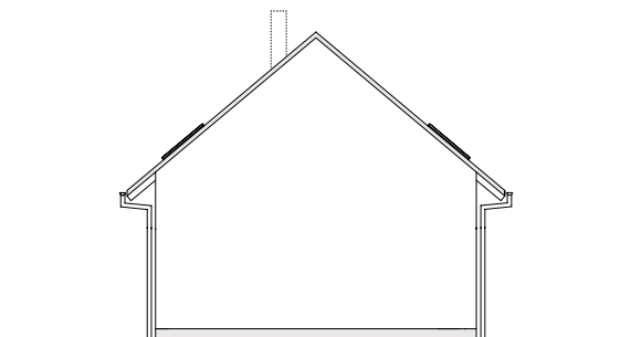
POHLED P3
