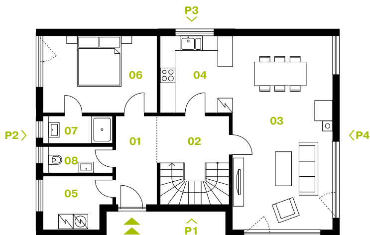
PŮDORYS PŘÍZEMÍ
